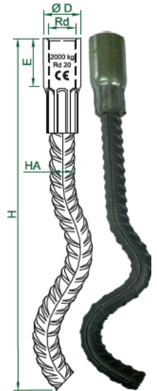
DOUILLE DE LEVAGE À ADHÉRENCE SINUS COURT/LONG
